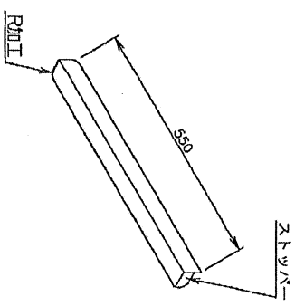
ホテルパンレール姿図
